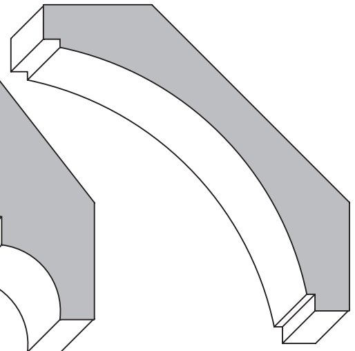
4032 3/4" x 3 1/4" Height - 2 5/16" Proj. - 2 5/16"
