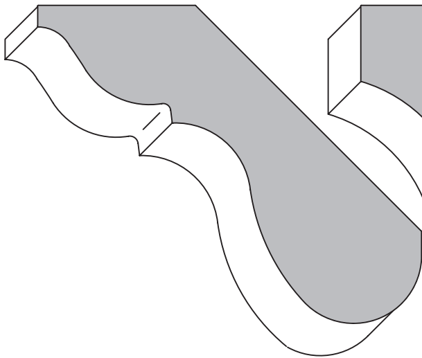
4024 1" x 3 1/2" Height - 2 3/8" Proj. - 2 7/8"
