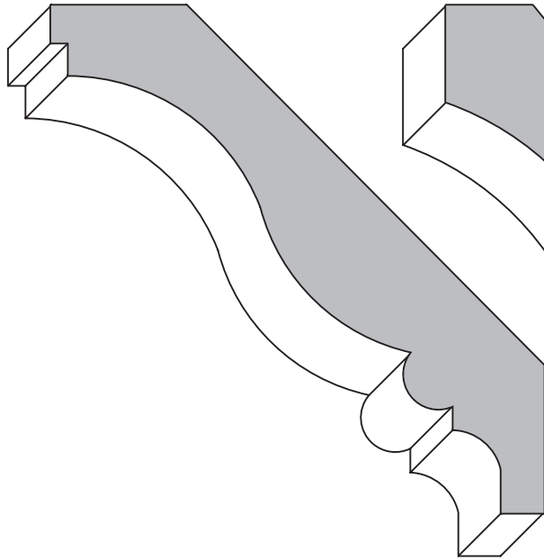
4033 3/4" x 4 1/8" Height - 2 15/16" Proj. - 2 7/8"
