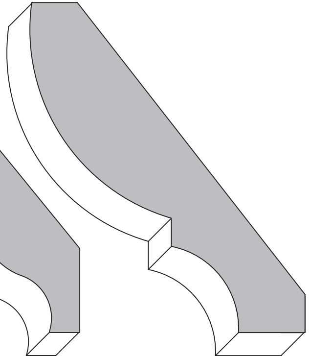
4008 3/4" x 4 3/8" Height - 3 1/2" Proj. - 2 5/8"
