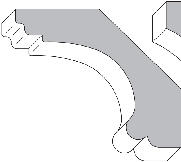
4023 1 1/4" x 3 7/8" Height- 2 1/2" Proj. - 3"
