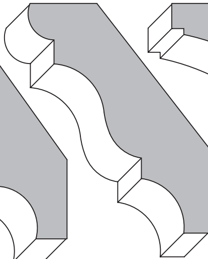
4002 3/4" x 3" Height - 2 3/8" Proj. - 1 13/16"
