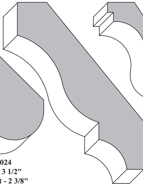
4004 3/4" x 3 5/8" Height - 2 7/8" Proj. - 2 3/16"
