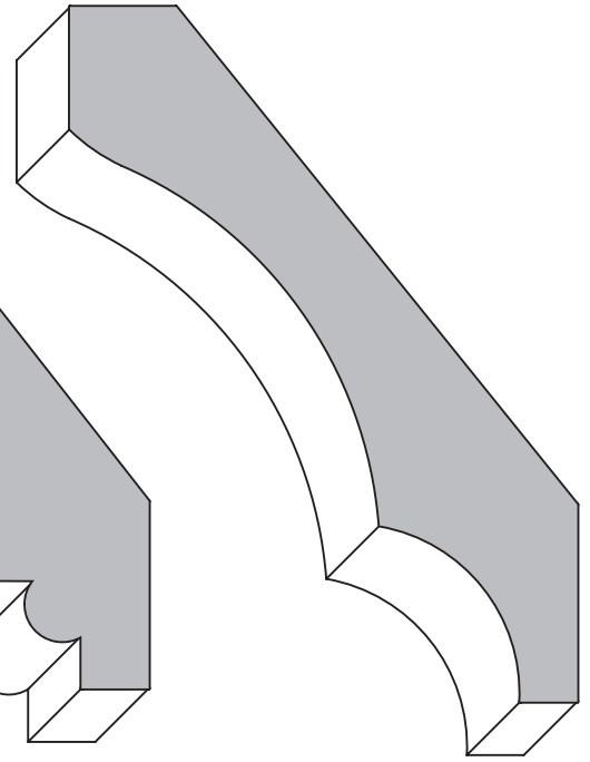
4006 3/4" x 4" Height- 3 3/16" Proj. - 2 7/16"
